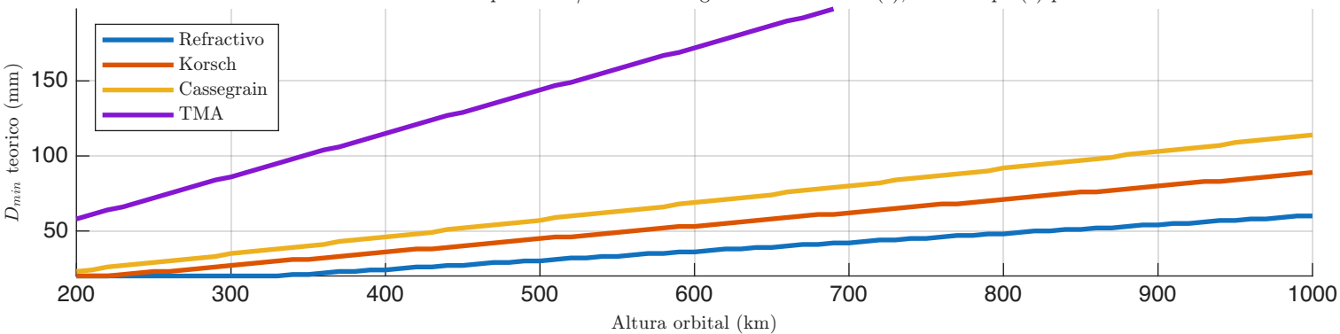
Detector 3: mínimo teórico por MTF/SNR - Configuración: 2 satélite(s), 2 telescopio(s) por satélite
